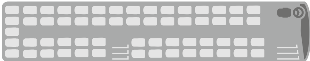
Variante 1 S 516 MD - 3 étoiles - porte centrale - 59 sièges
