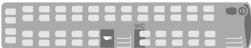
Variante 2 S 516 HD - 4 étoiles - 48 sièges - classe 3 + WC + cuisine de bord
