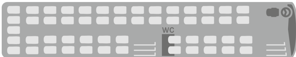
Variante 1 S 516 HD - 3 étoiles - 53 places assises + WC
